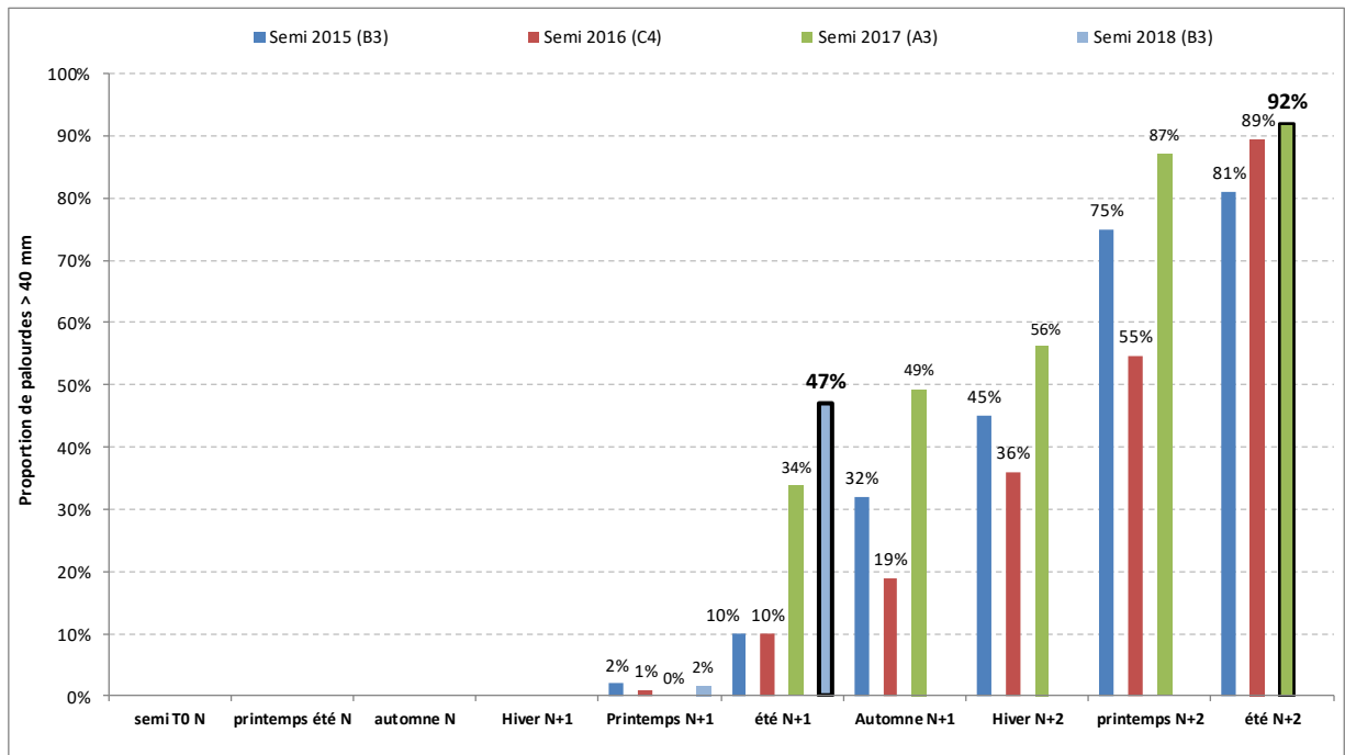
Evolution de la proportion de palourdes de taille > 40 mm
