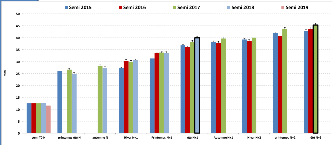
Evolution de la taille des palourdes sur un cycle entier d'élevage
